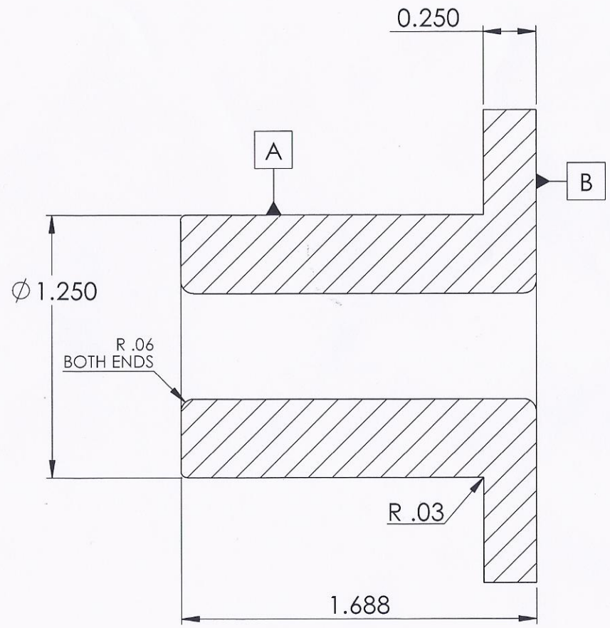
SECTION A-A SCALE 2 : 1.3
